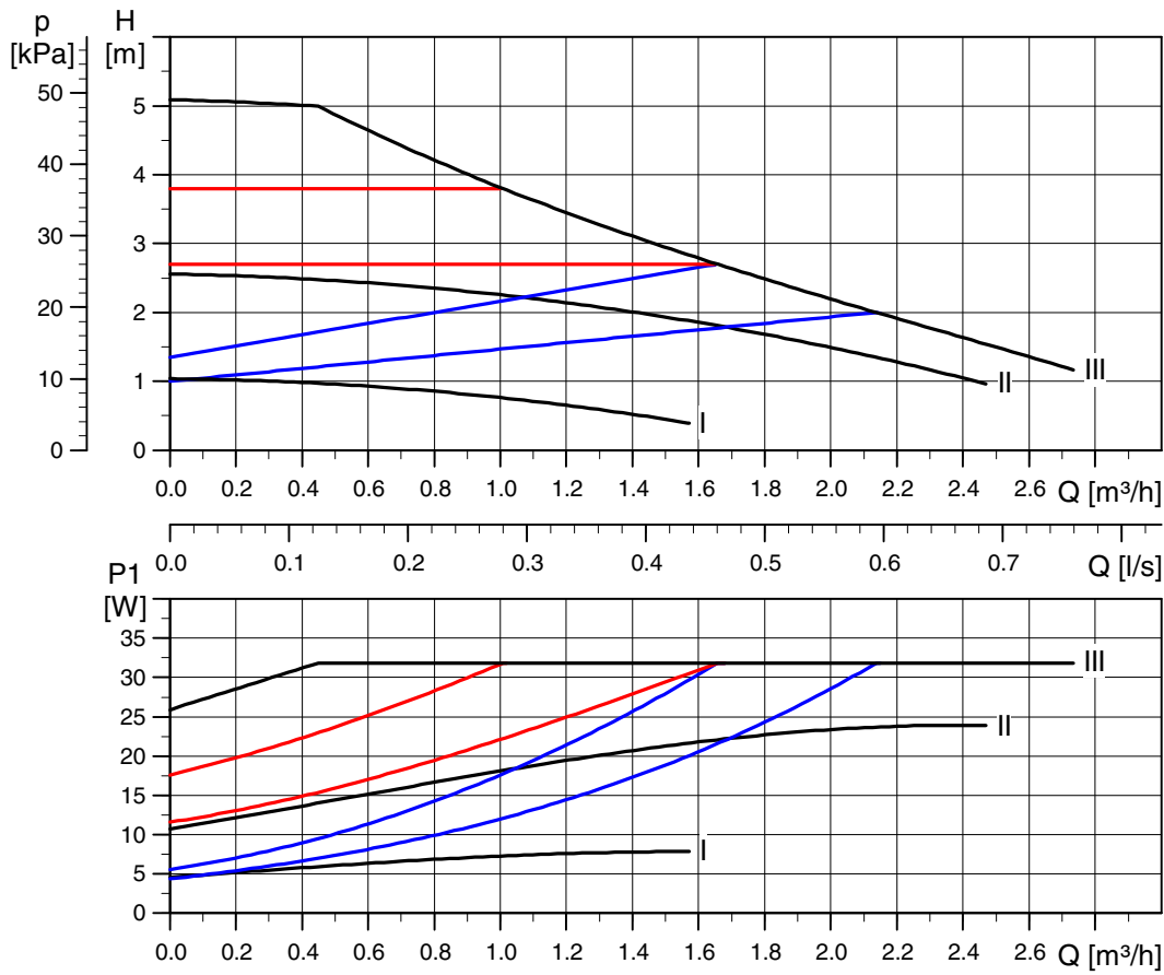
Fig. 20 Curbe caracteristiche, ALPHA2 L XX-50
